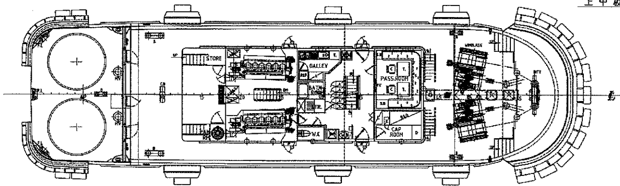
上甲板上
